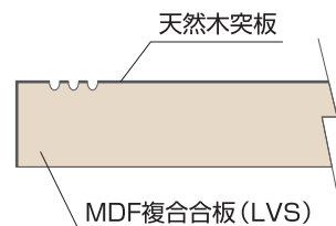
● 踏板断面図 (すべり止め3本U溝加工)
